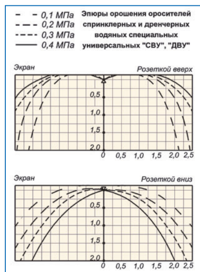
Рис. 2. Универсальные оросители СВУ, ДВУ
