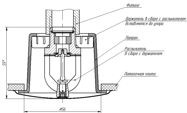
б) комплект для скрытого монтажа ДАЭ 100.432.000 совместно с распылителем
