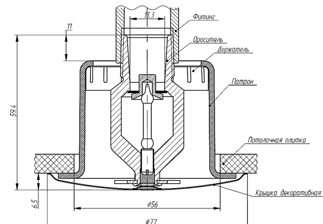
а) комплект для скрытого монтажа ДАЭ 100.435.000 совместно с оросителем
