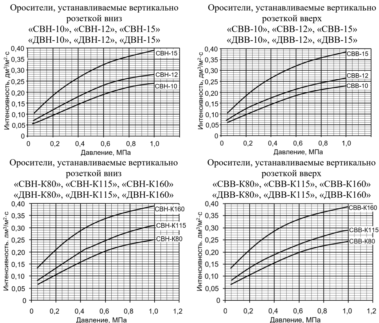
Рисунок 2 – Эпюры зависимости средней интенсивности орошения от давления
