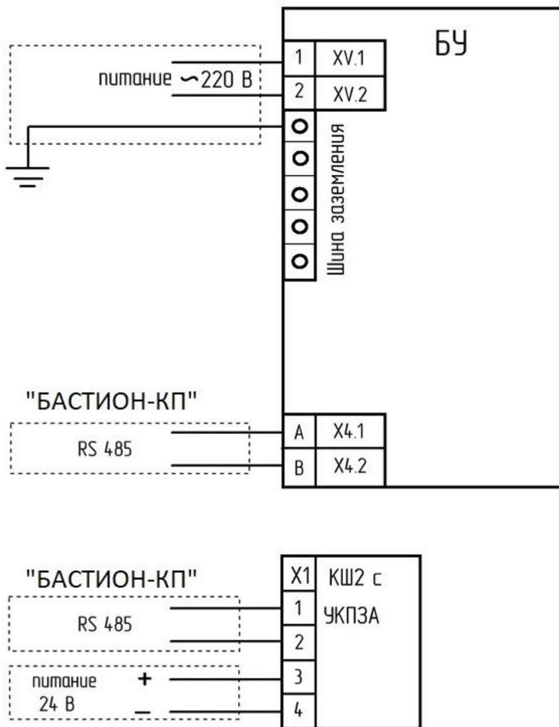
Рисунок В.1 – Схема подключения
