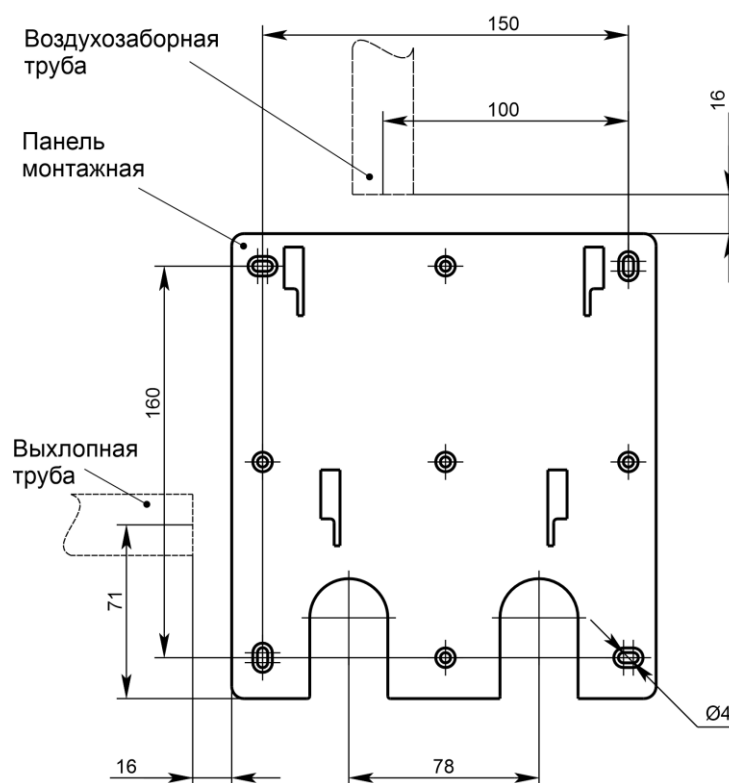
Рисунок 9 – Установочные размеры монтажной панели
