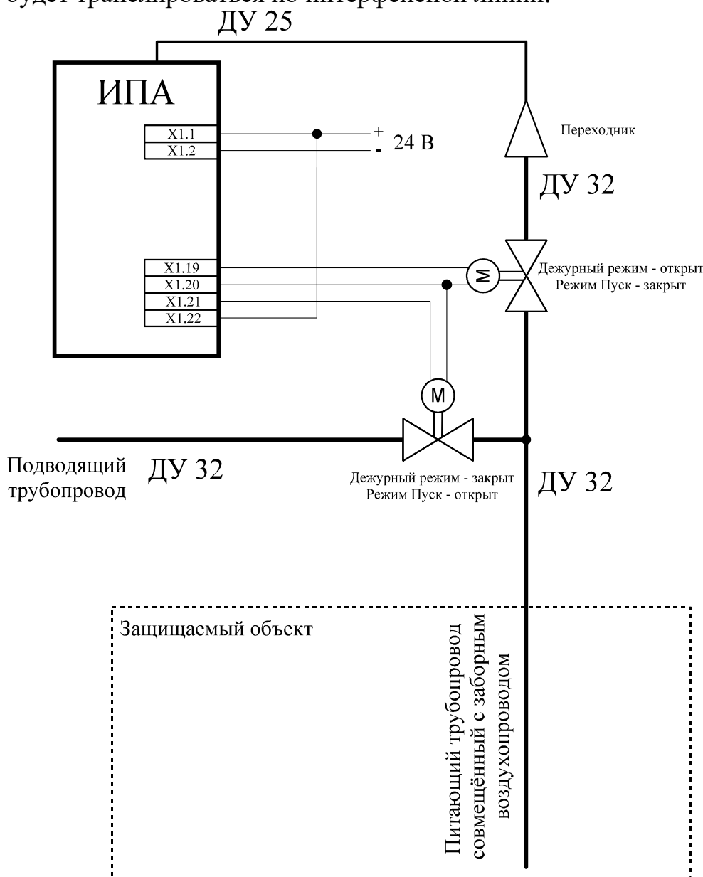
Рисунок 6 – Схема подключения Извещателя с управлением кранами. Вариант 1
