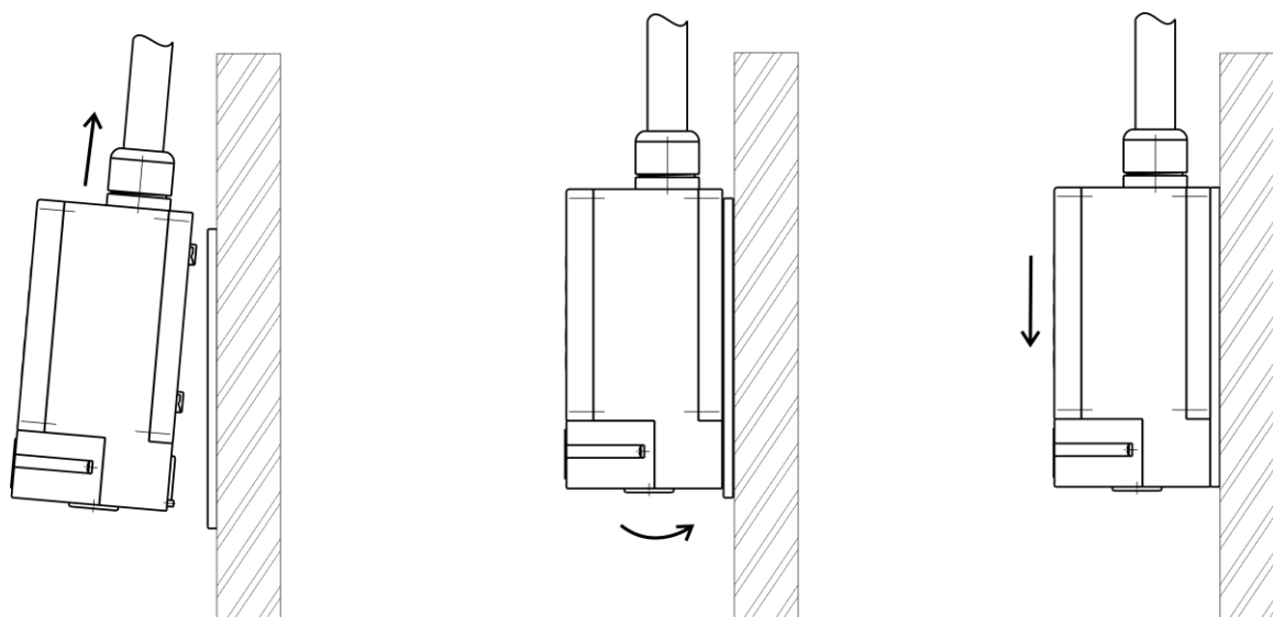
Рисунок 11 – Установка Извещателя на монтажную панель
