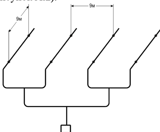
Рисунок А.2 – Пример конфигурации трубопровода Извещателя для алгоритма А
