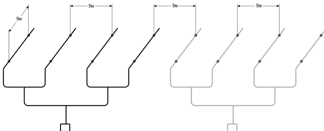
Рисунок А.3 – Пример конфигурации трубопровода Извещателя для алгоритма В
