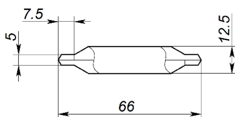
Рисунок 13 – Рекомендуемый тип сверла – центровочное сверло 2317-0106 ГОСТ 14952-75 (поставляется по требованию потребителя)
