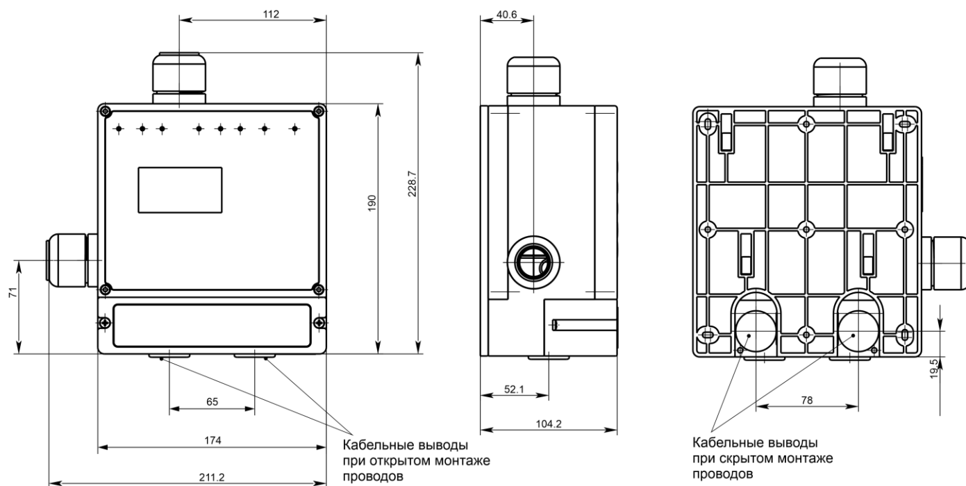
Рисунок 10 – Габаритные и присоединительные размеры Извещателя
