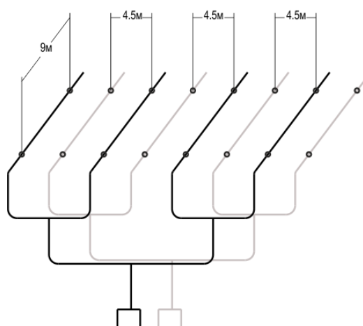
Рисунок А.4 – Пример конфигурации трубопровода извещателя для алгоритма С
