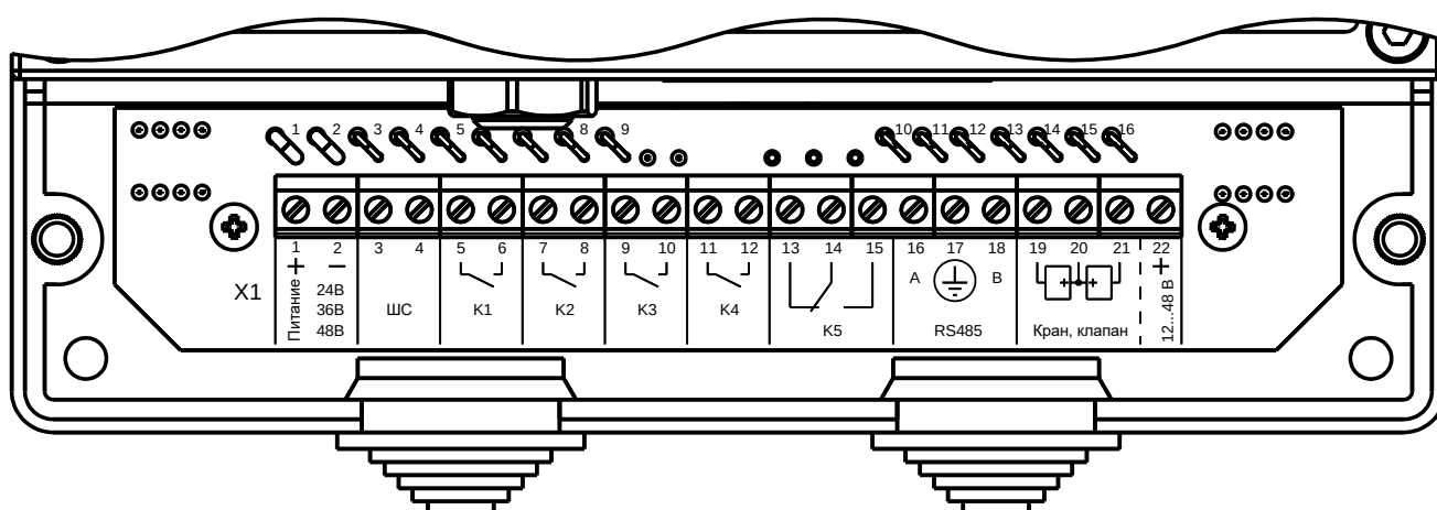
Рисунок 15 – Клеммы Извещателя
