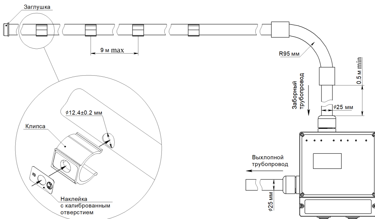
Рисунок 12 – Подключение воздухозаборной системы
