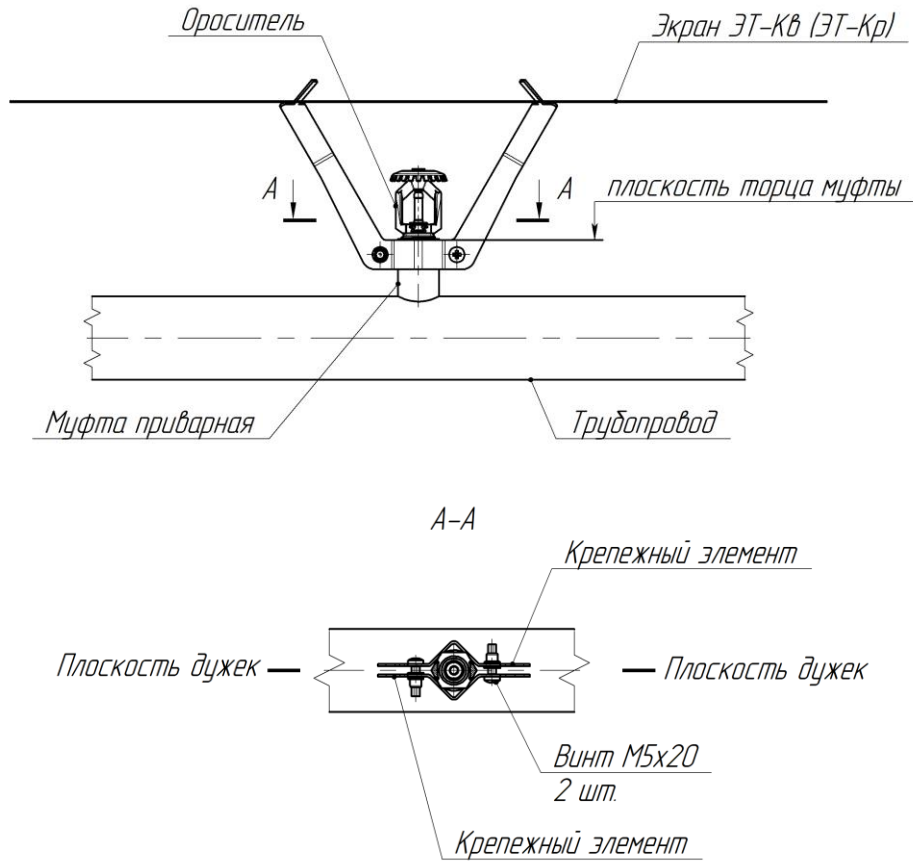
Рисунок 5 – Схема положения экрана относительно оросителя монтажным положением вертикально вверх
