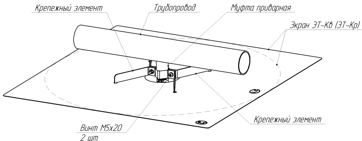
Рисунок 1 – Схема установки экрана на муфту приварную для оросителя (распылителя) монтажным положением вертикально вниз
