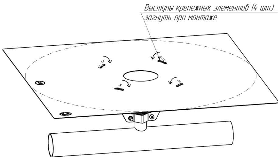
Рисунок 6 – Схема фиксации экрана с крепежными элементами для оросителя (распылителя) монтажным положением вертикально вверх
