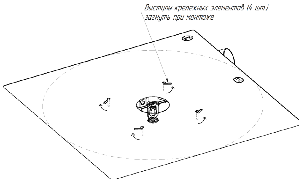
Рисунок 2 – Схема фиксации экрана с крепежными элементами для оросителя (распылителя) монтажным положением вертикально вниз
