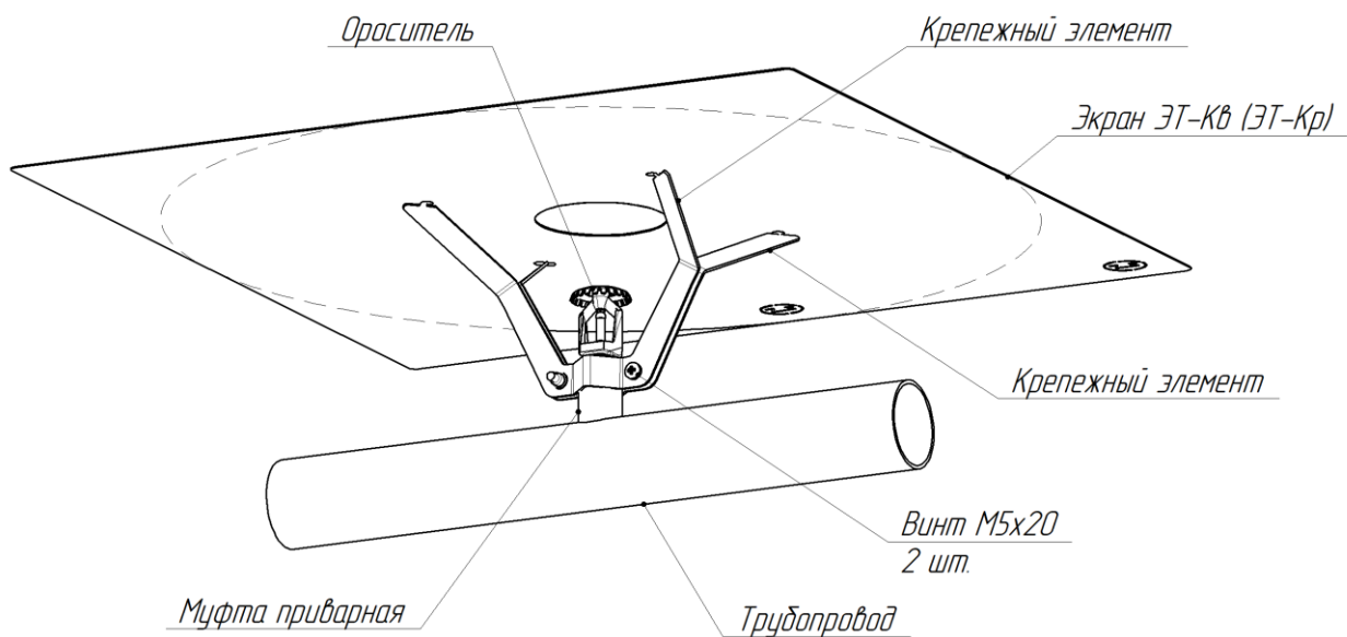
Рисунок 4 – Схема установки экрана на муфту приварную для оросителя монтажным положением вертикально вверх
