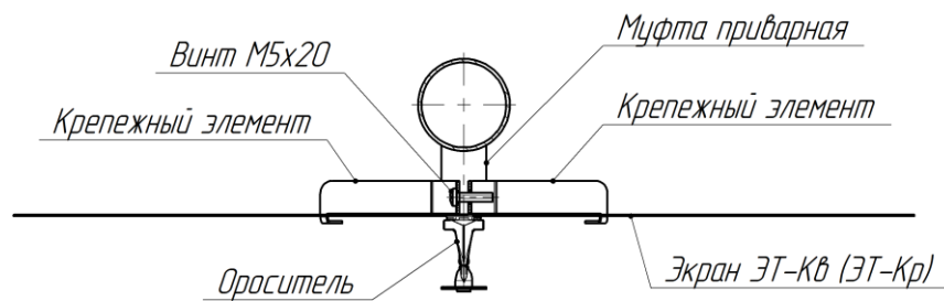
Рисунок 3 – Схема положения экрана относительно оросителя (распылителя) монтажным положением вертикально вниз
