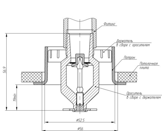
а) устройство углубленного монтажа ДАЭ 100.285.000 совместно с оросителем установленным вертикально вниз
