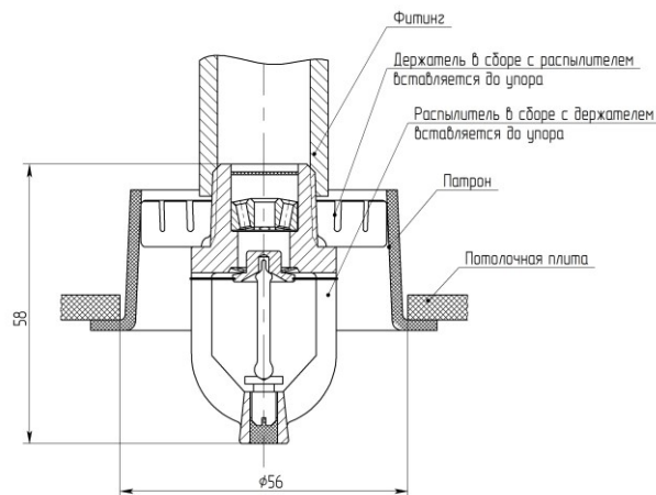
б) устройство углубленного монтажа ДАЭ 100.285.000 совместно с распылителем установленным вертикально вниз
