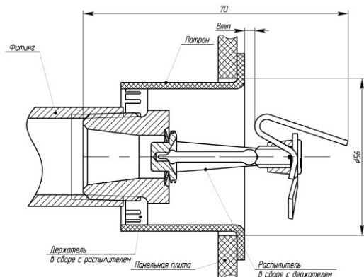
в) устройство углубленного монтажа ДАЭ 100.285.000 совместно с оросителем установленным горизонтально
