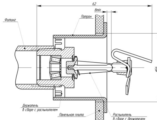
г) устройство углубленного монтажа ДАЭ 100.285.000 совместно с распылителем установленным горизонтально
