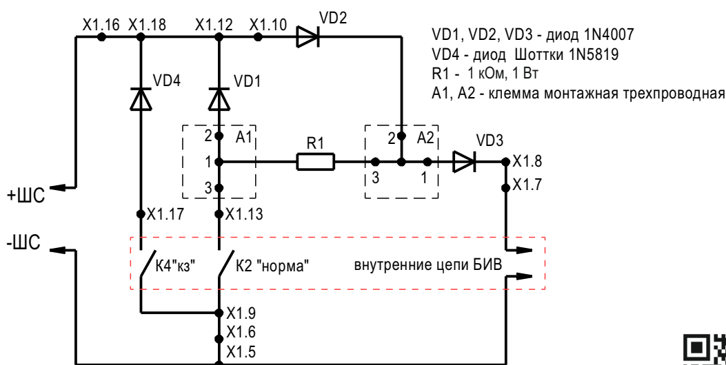
Схема электрическая принципиальная подключения БИВ
