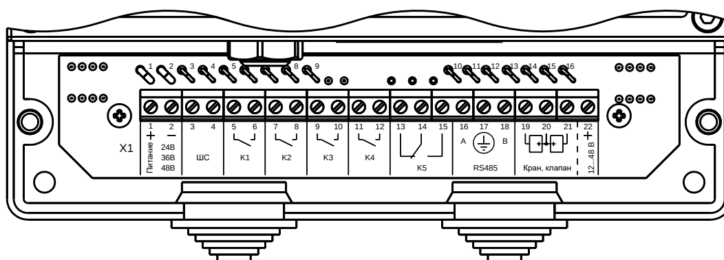
Рисунок 15 – Клеммы Извещателя
