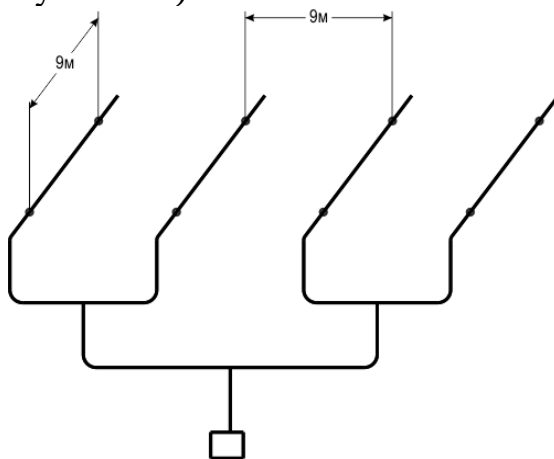
Рисунок А.2 – Пример конфигурации трубопровода ИПА для алгоритма А
