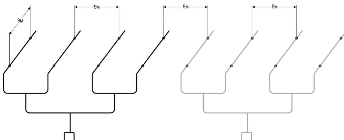
Рисунок А.3 – Пример конфигурации трубопровода ИПА для алгоритма В
