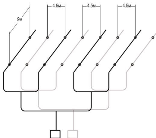
Рисунок А.4 – Пример конфигурации трубопровода ИПА для алгоритма С
