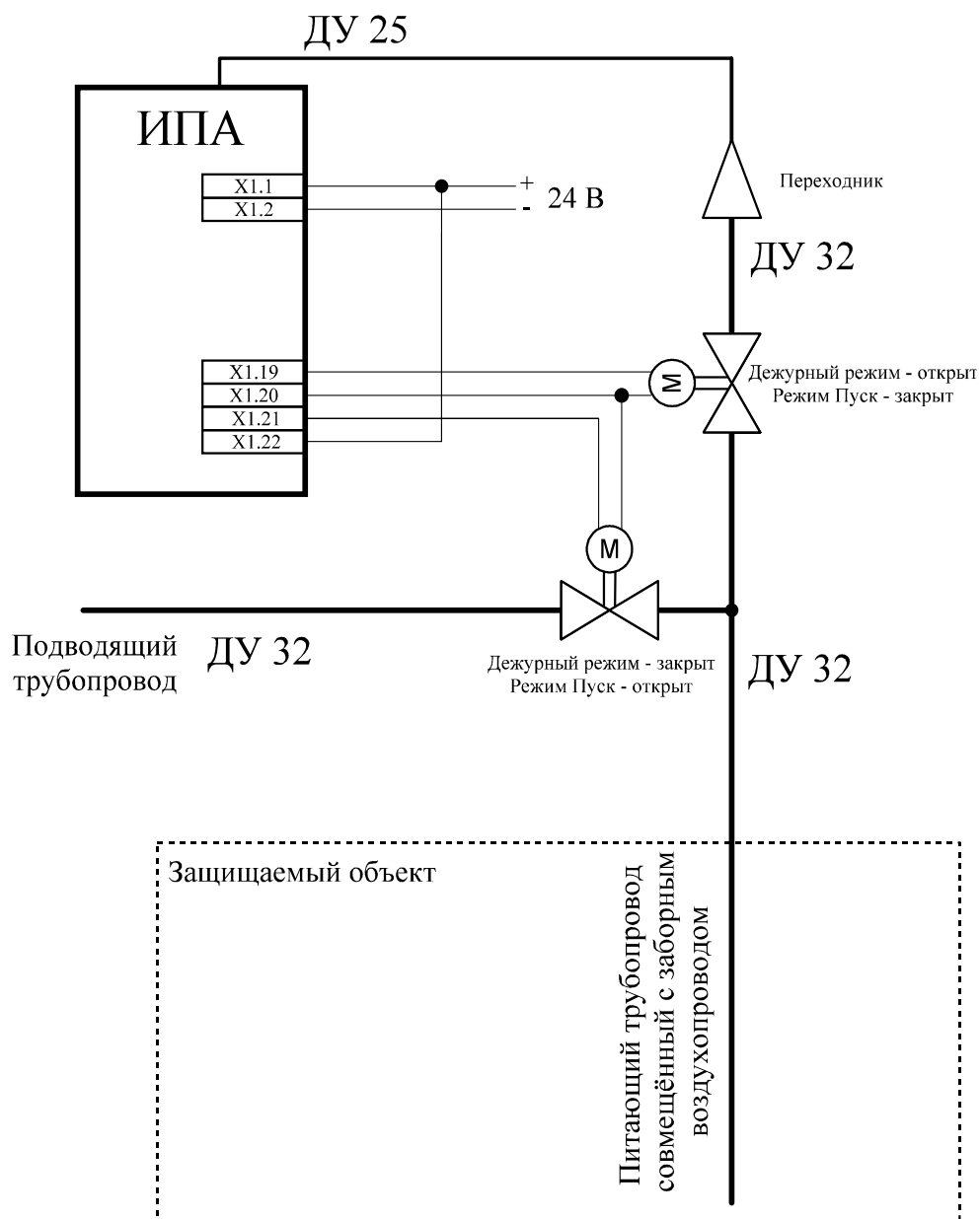
Рисунок 6 – Схема подключения извещателя с управлением кранами. Вариант 1
