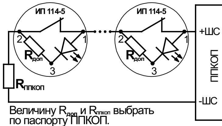
Схема подключения ИП 114-5 в шлейф ППКОП
