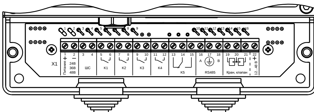
Рисунок 15 – Клеммы извещателя
