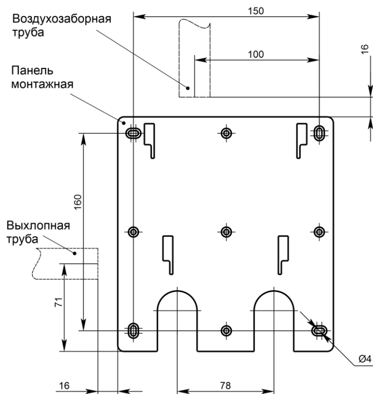
Рисунок 9 – Установочные размеры монтажной панели
