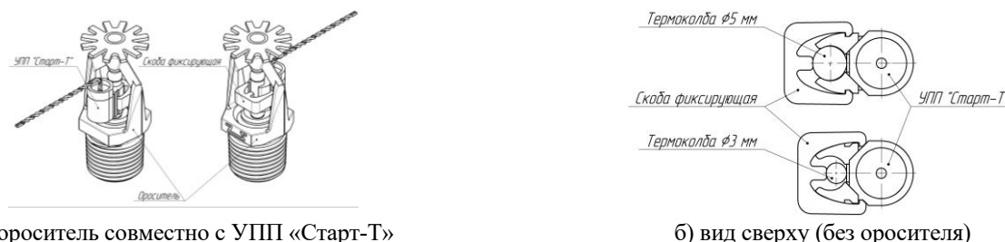
Рисунок 1 – Схема установки УПП «Старт-Т» на спринклерный ороситель
