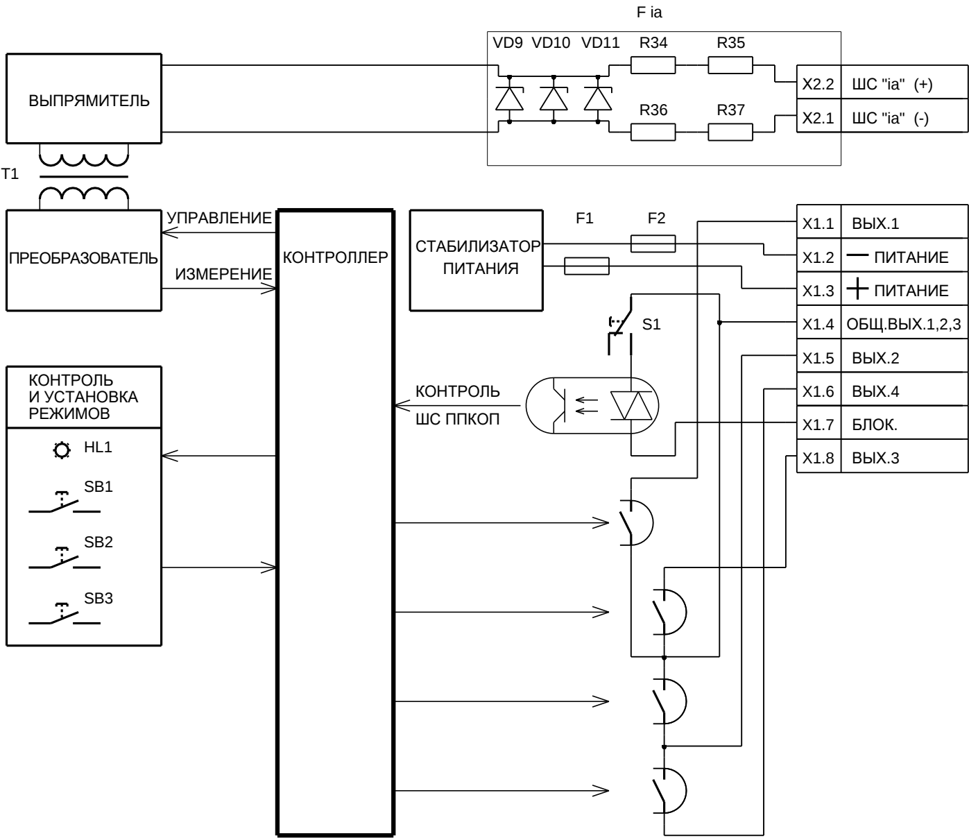
Рисунок Г.1 – Схема электрическая функциональная БИВ УПКОП 135-1-1
