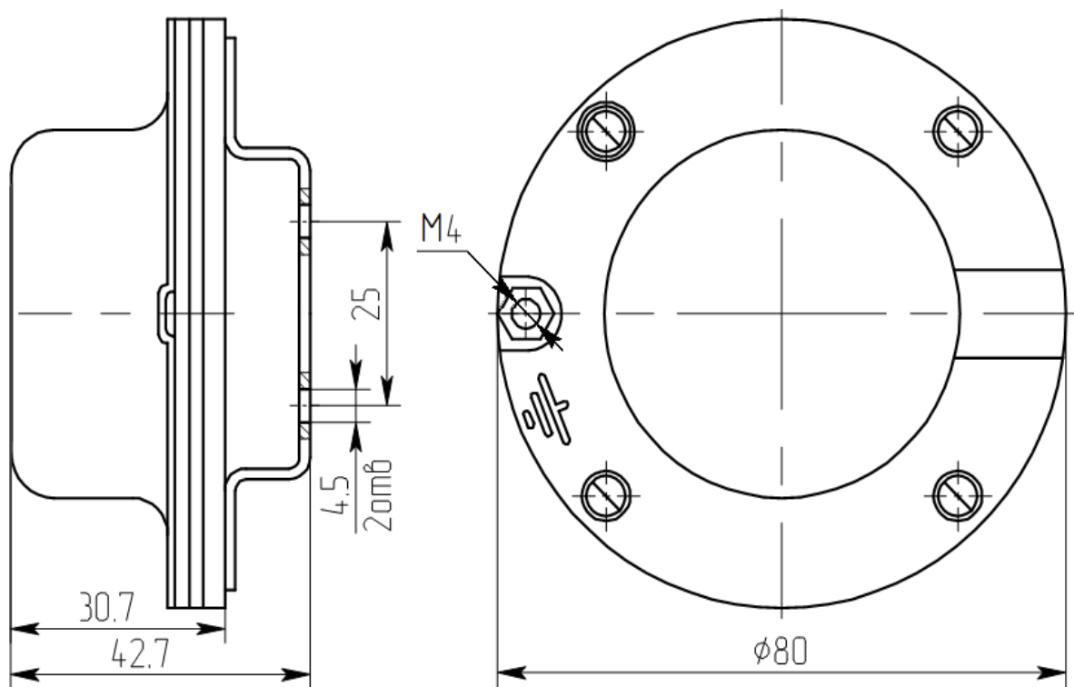
Рисунок В.2 – Габаритные и установочные размеры выносного элемента ЭВ
