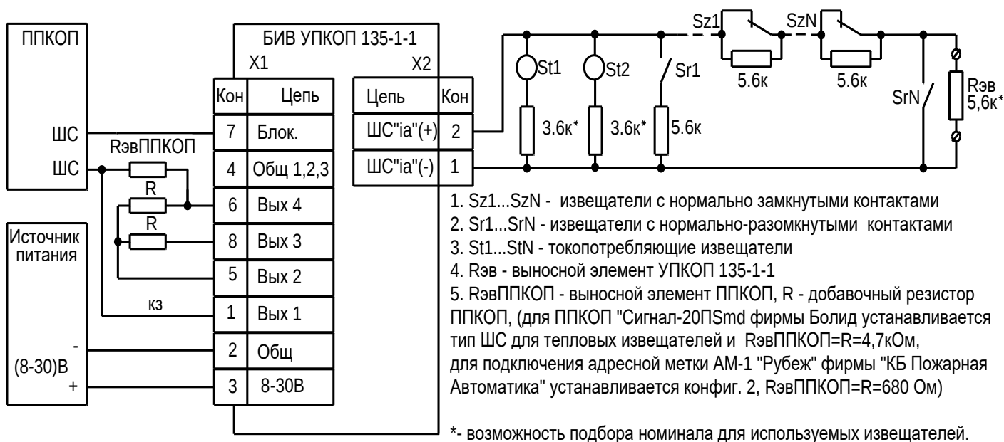
Рисунок Д.1 – Типовая схема подключения устройства УПКОП 135-1-1 к ППКОП
