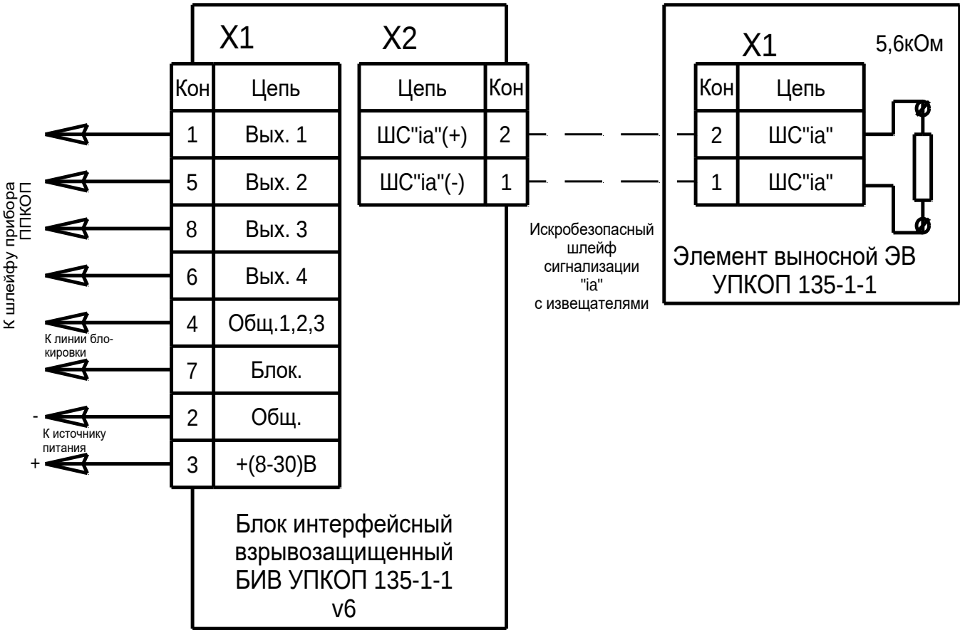
Рисунок А.1 – Схема электрическая соединений УПКОП 135-1-1
