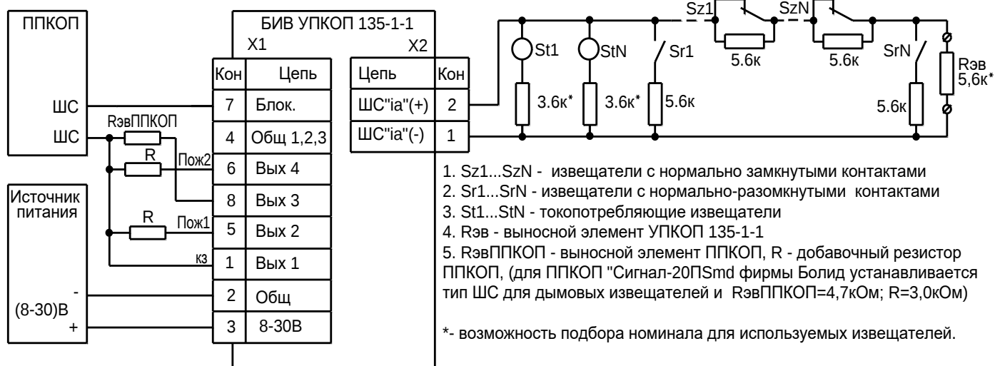
Рисунок Д.1 – Типовая схема подключения устройства УПКОП 135-1-1 к ППКОП
