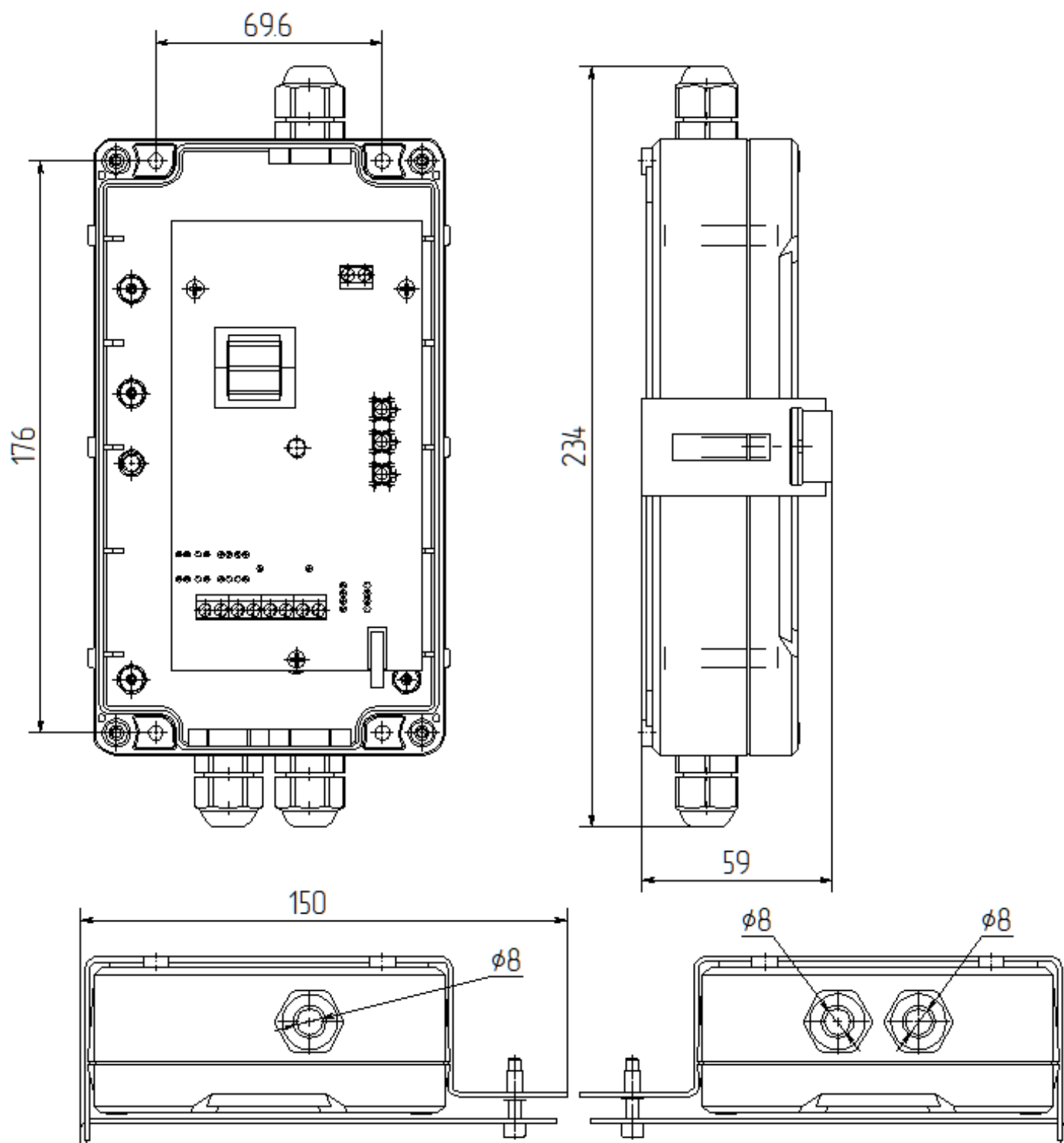
Рисунок В.1 – Габаритные и установочные размеры блока БИВ
