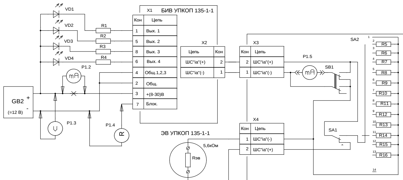
Рисунок Б.1 – Схема подключения УПКОП 135-1-1 для проверки его технического состояния
