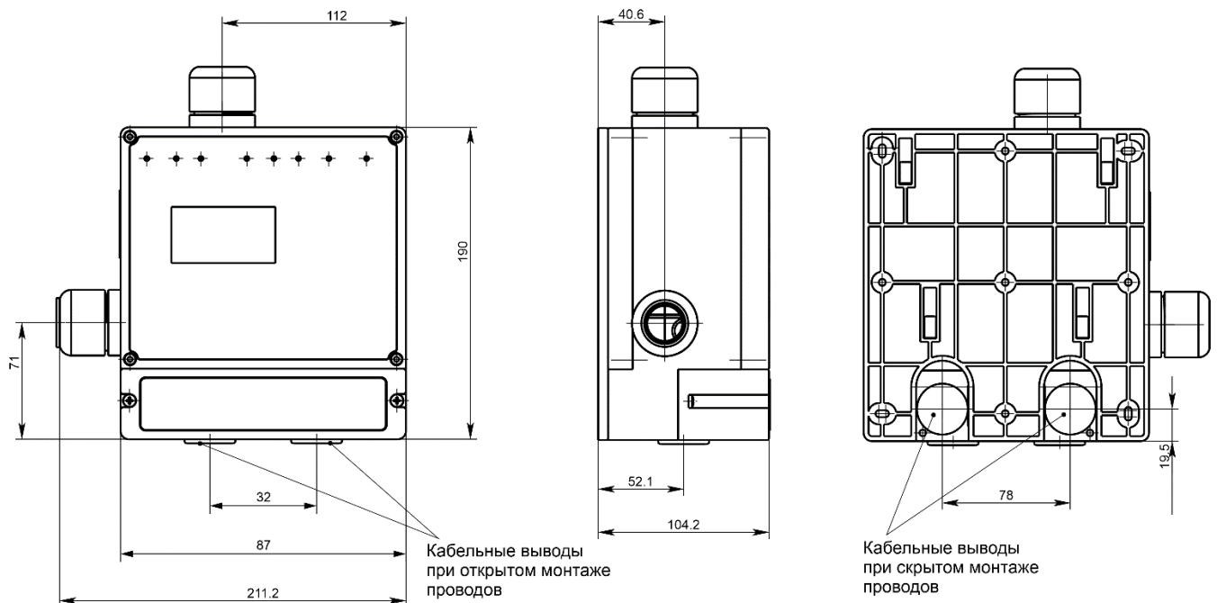
Рисунок 10 – Габаритные и присоединительные размеры извещателя
