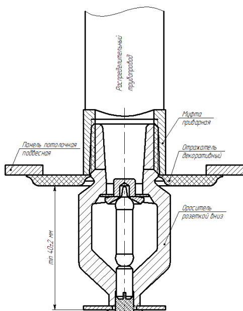
а) отражатель декоративный ДАЭ 100.210.001-01 совместно с оросителем розеткой вниз
