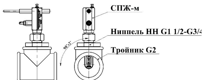
Рисунок А.4 – DN 50
