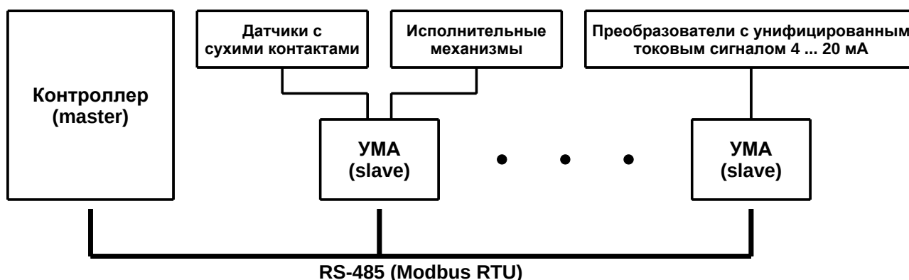
Рисунок 1.1 – Функциональная схема сети RS-485
