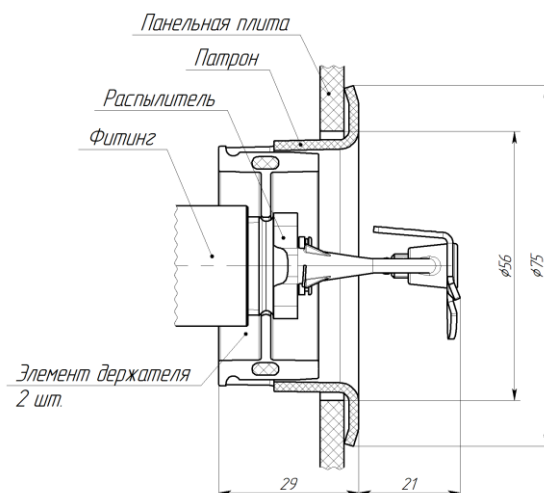
г) устройство углубленного монтажа ДАЭ 100.285.000 совместно с распылителем установленным горизонтально
