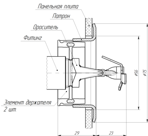
а) устройство углубленного монтажа ДАЭ 100.285.000 совместно с оросителем установленным вертикально вниз
