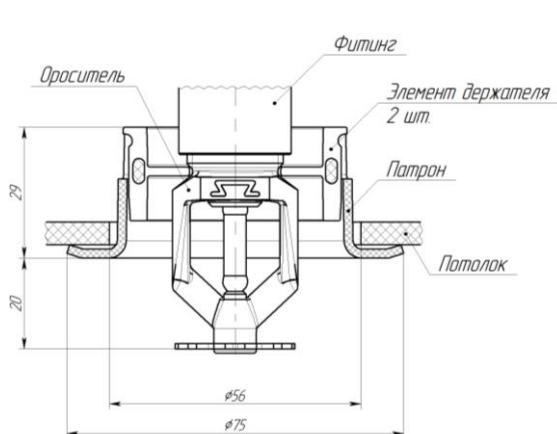
а) устройство углубленного монтажа ДАЭ 100.285.000 совместно с оросителем установленным вертикально вниз
