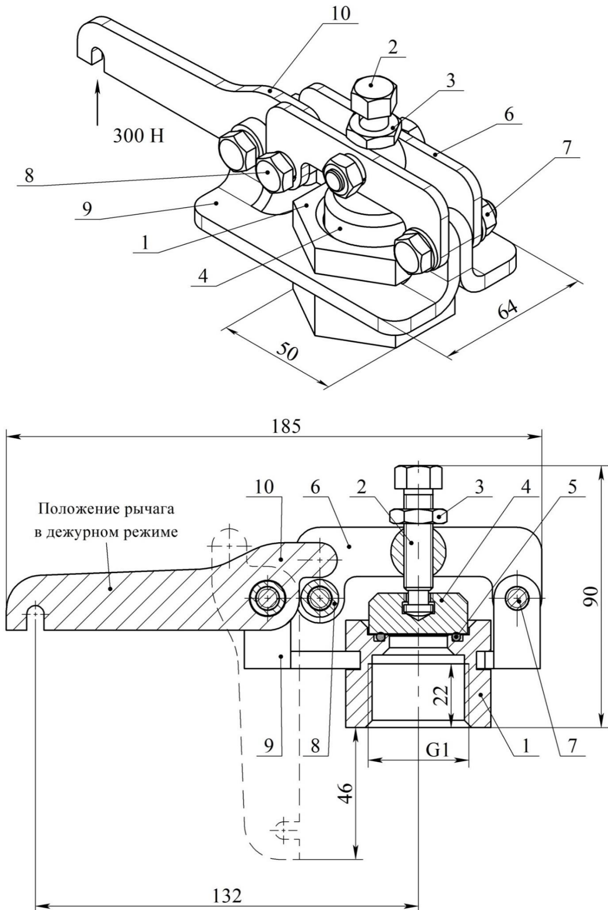
Рисунок 1 – Клапан побудительный тросовый "КПТА-25"
