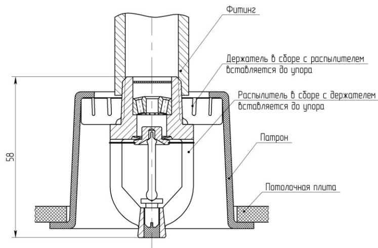
Рисунок 1 – Устройство углубленного монтажа ДАЭ 100.285.000 совместно с распылителем
