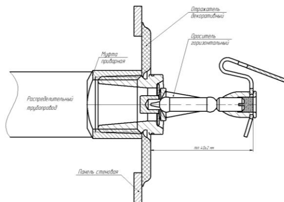
б) отражатель декоративный ДАЭ 100.210.001-01 совместно с горизонтальным оросителем
