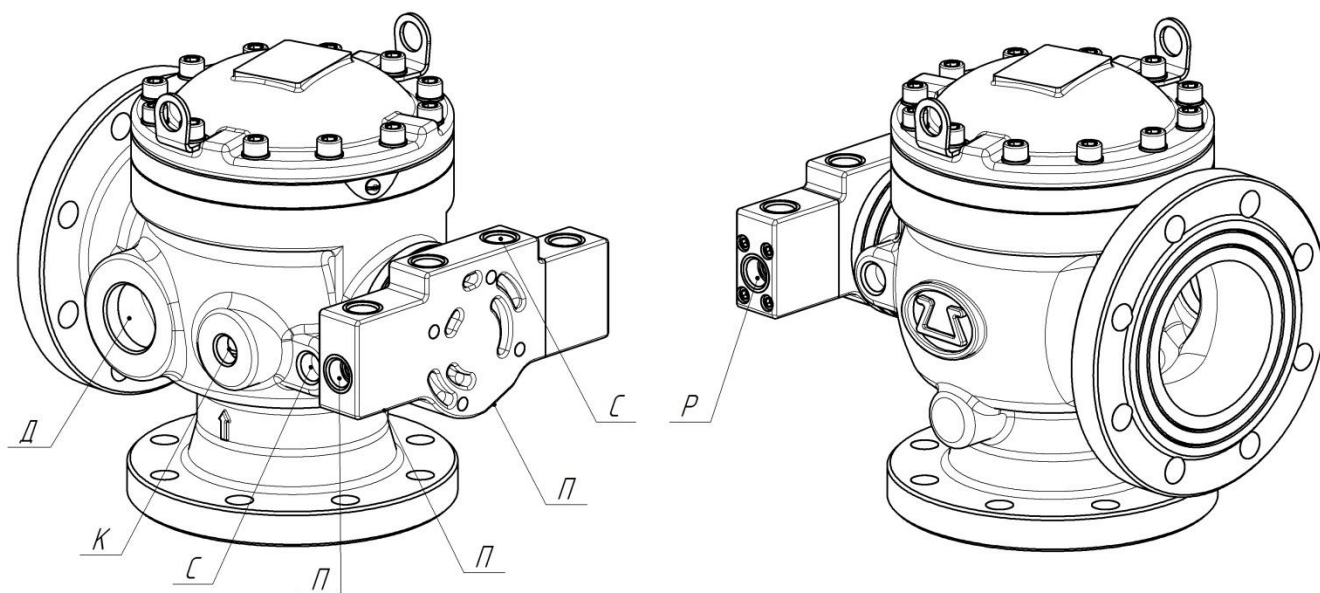
Рисунок 2 – Клапан мембранный универсальный КСД типа КМУ. Общий вид «Д» – отверстие дренажное, «К» – отверстие контрольное, «П» – отверстие побудительное, «С» – отверстие сигнальное, «Р» – отверстие рабочее
