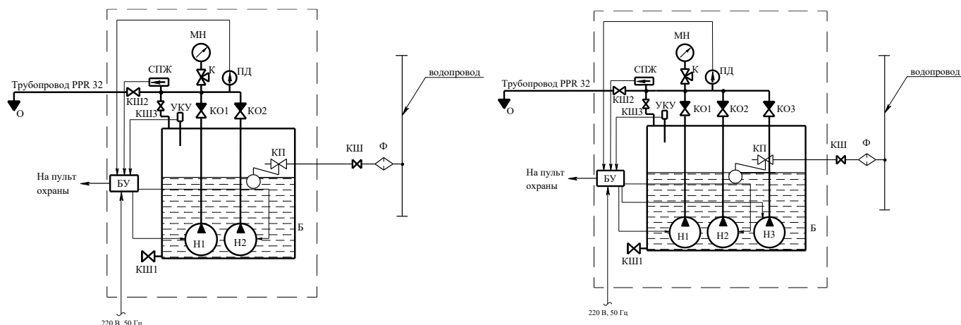
Рисунок 3—Схема функциональная системы спринклерного пожаротушения на основе МПОВ 500.3 (пример)
