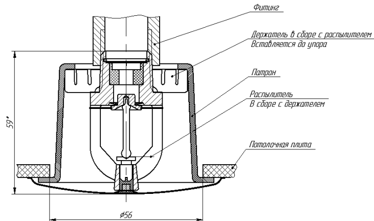
Рисунок 1 – Комплект для скрытого монтажа ДАЭ 100.432.000 совместно с распылителем
