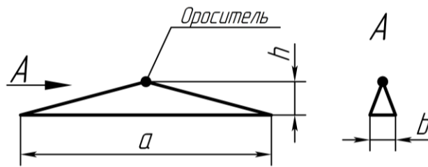
Рисунок 2 – Карта орошения Оросителя «ЗВН-180»
