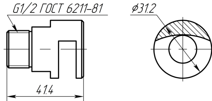
Рисунок 1 – Ороситель «ЗВН-180»
