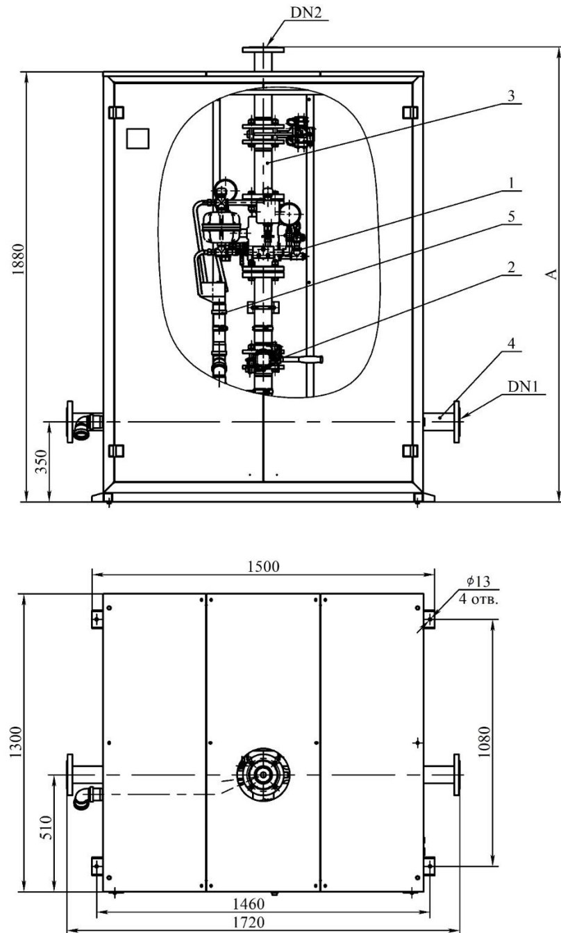
Рисунок 1 – Общий вид и состав шкафа для размещения узла управления группы «С»
