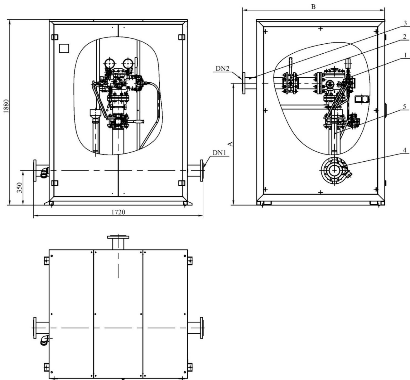
Рисунок 2 – Общий вид и состав шкафа для размещения узла управления группы «СД»
