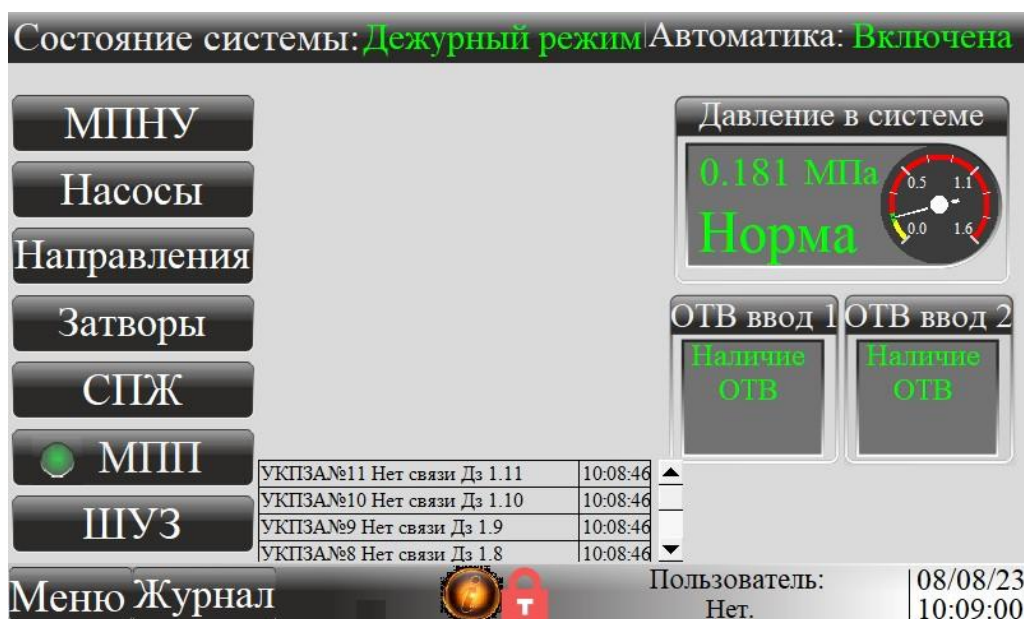
Рисунок 1 – Главный экран ШУК
