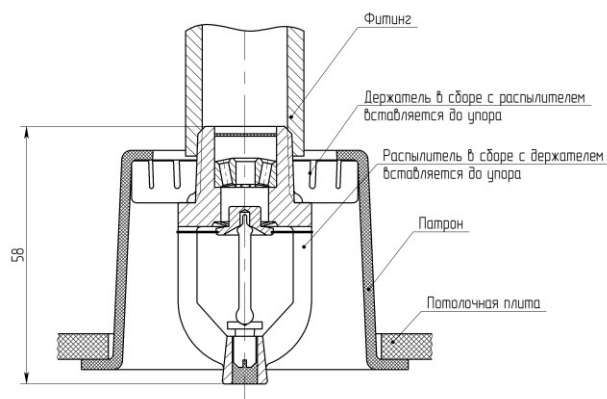
б) устройство углубленного монтажа ДАЭ 100.285.000 совместно с распылителем
