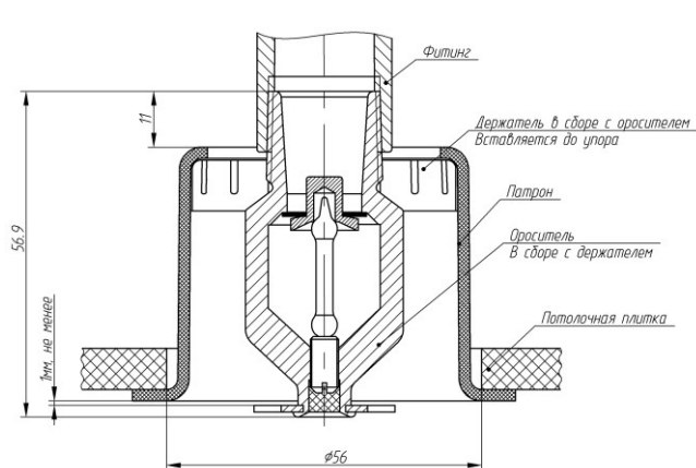
а) устройство углубленного монтажа ДАЭ 100.285.000 совместно с оросителем
